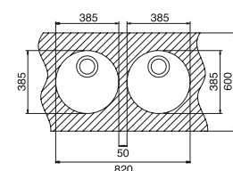
MIN. BASE UNIT: 90
